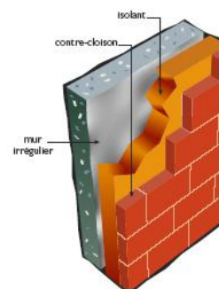
Bloc maçonné/contre cloison
