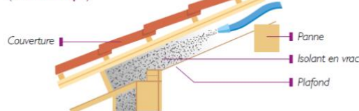
L'isolation par insufflation (vue en coupe)
